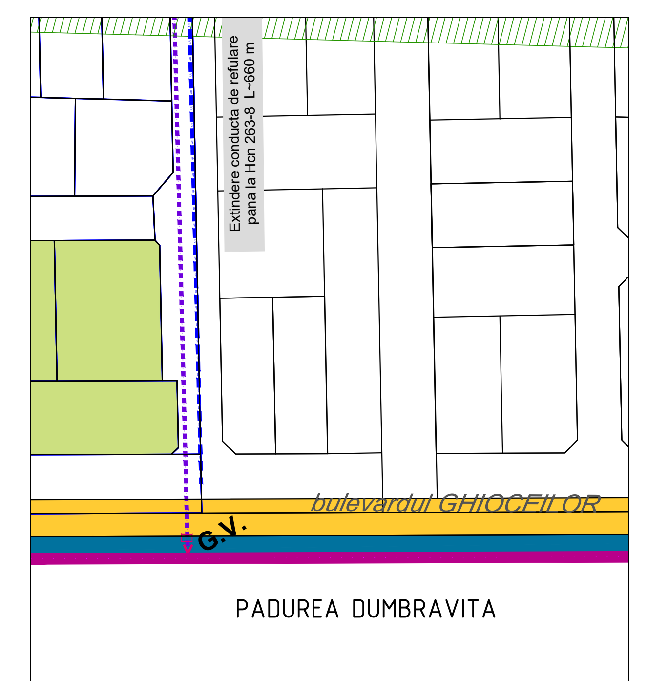
Detalii de evacuare ape pluviale in canal ANIF scara 1:1000
