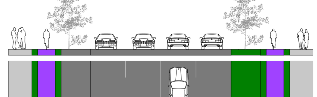
Secțiune AA"
