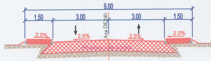
PROFIL TRANSVERSAL TIP se aplica pe DE240 Scara 1:100
