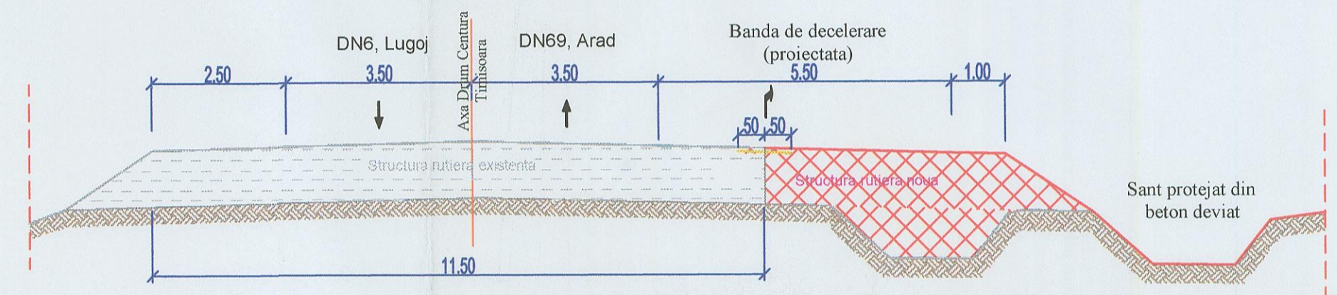
SECTIUNE TRANSVERSALA A-A ETAPA I se aplica pe drum Centura Timisoara Scara 1:100
