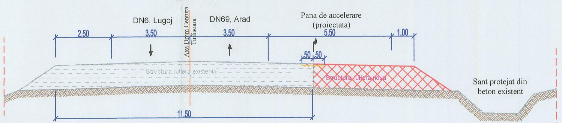
SECTIUNE TRANSVERSALA B-B ETAPA I se aplica pe drum Centura Timisoara Scara 1:100
