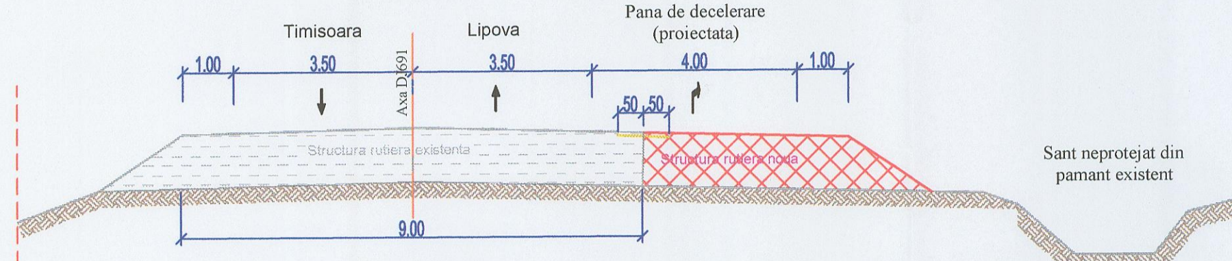
SECTIUNE TRANSVERSALA C-C ETAPA I se aplica pe DJ691 Scara 1:100
