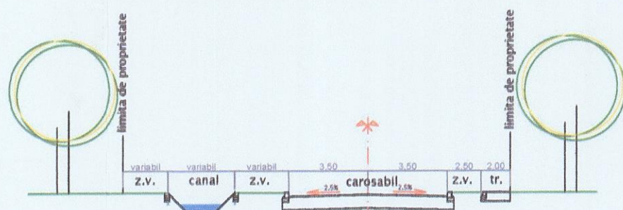
PROFIL TRANSVERSAL TIP PTT 1
