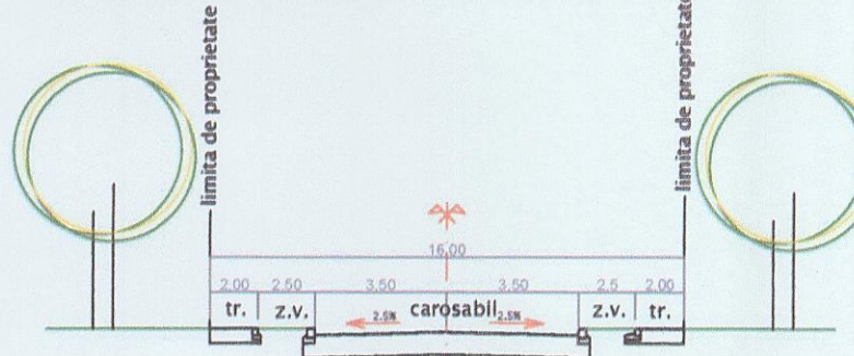
PROFIL TRANSVERSAL TIP PTT 2
