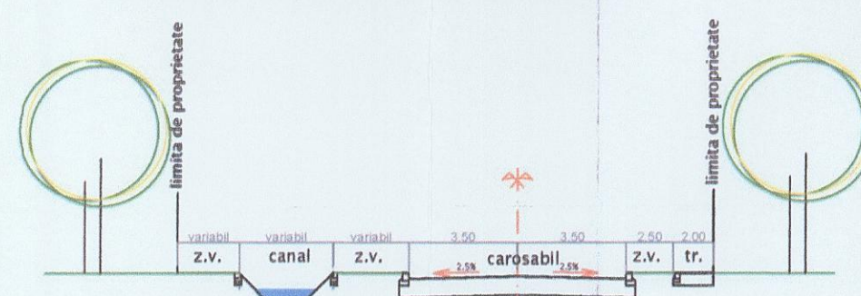
PROFIL TRANSVERSAL TIP PTT 1
