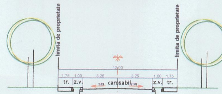
PROFIL TRANSVERSAL TIP PTT 3
