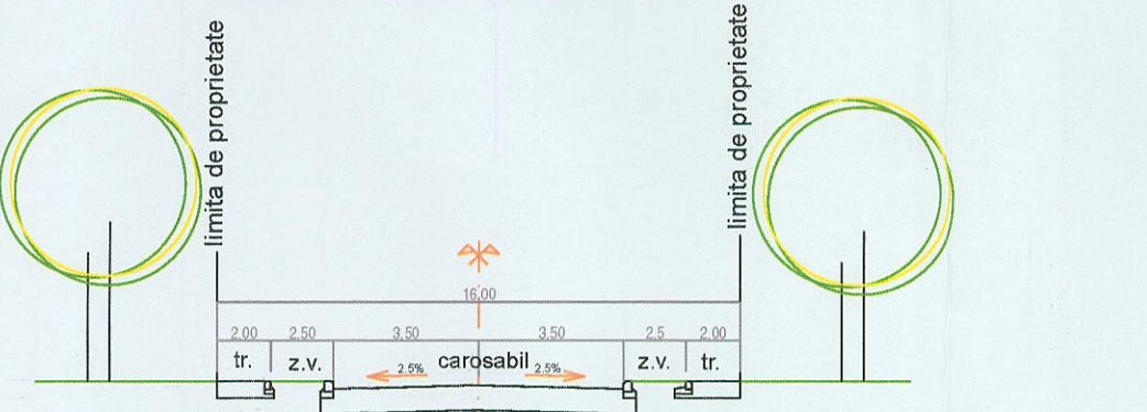
PROFIL TRANSVERSAL TIP PTT 2
