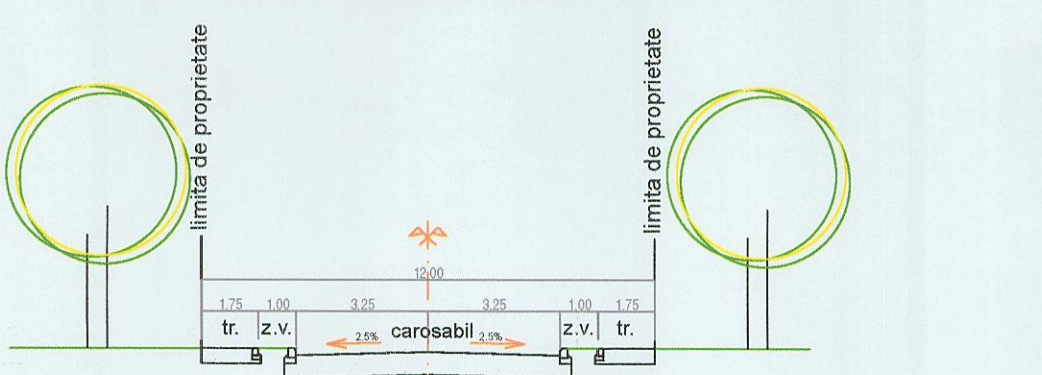
PROFIL TRANSVERSAL TIP PTT 3
