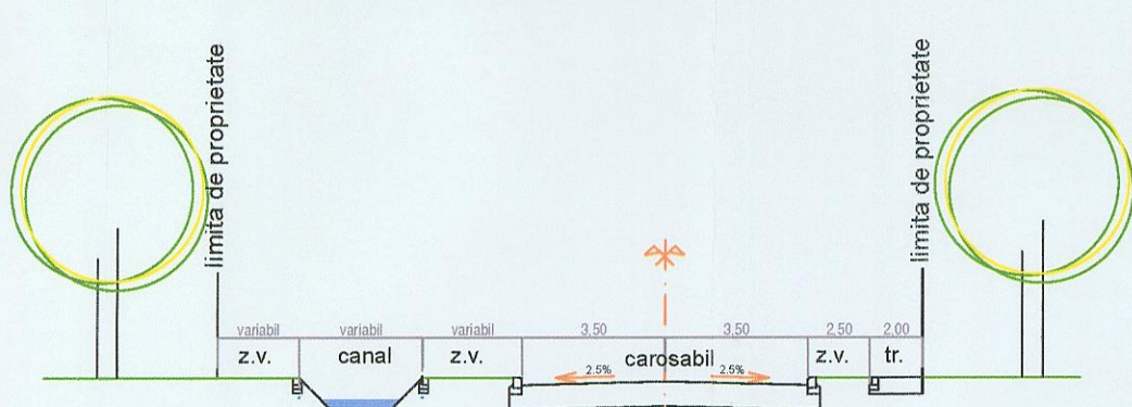
PROFIL TRANSVERSAL TIP PTT 1
