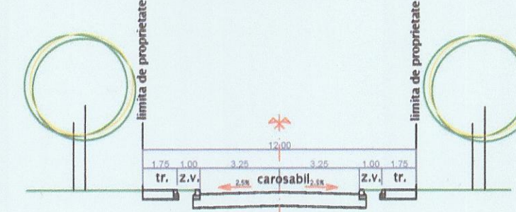
PROFIL TRANSVERSAL TIP PTT 3
