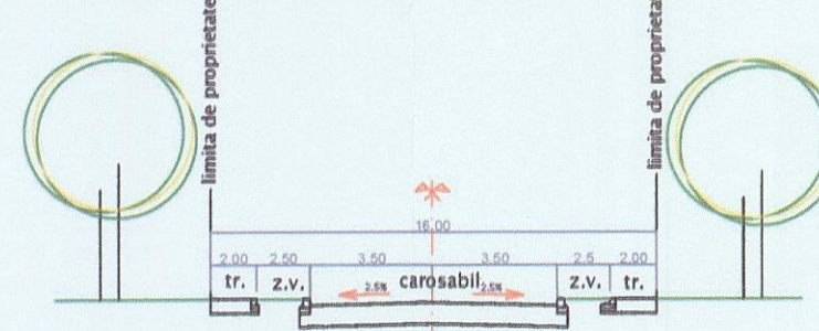
PROFIL TRANSVERSAL TIP PTT 2
