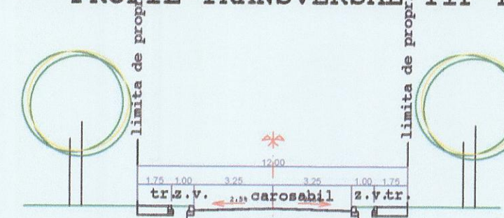
PROFIL TRANSVERSAL TIP PTT
