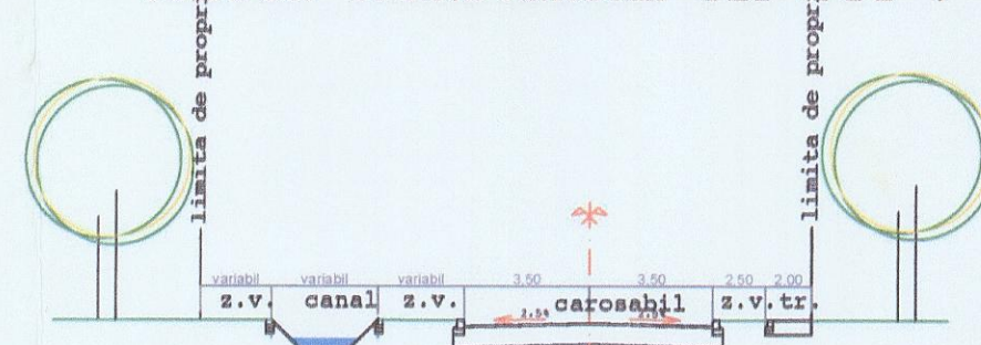
PROFIL TRANSVERSAL TIP PTT 1
