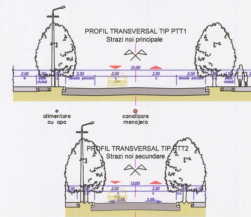
PROFILI STRAZI - SC. 1:200
