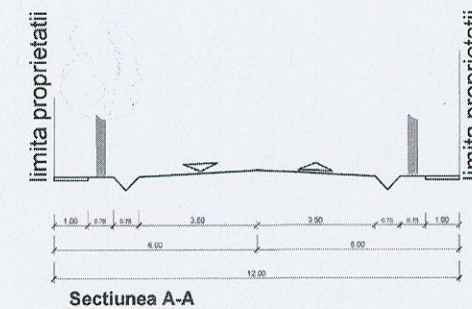
PROFILI TRANSVERSALE scara 1 : 100
