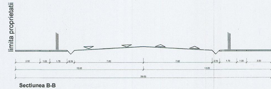
PROFILI TRANSVERSALE scara 1 : 100
