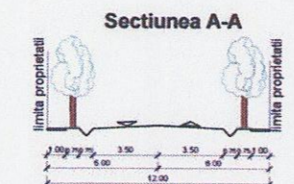
PROFIL TRANSVERSAL scara 1 : 200
